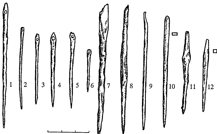
13 pav. Adatos (1–6) ir ylos (7–12): 1 – kapas Nr. 225 (EM 2:916), 2–5 – atsitiktinės (EM 2:1872–1875), 6 – kapas Nr. 359 (EM 2:1301), 7 – kapas Nr. 190 (EM 2:577), 8 – kapas Nr. 361 (EM 2:2218), 9 – kapas Nr. 310 (EM 2:684), 10–12 – atsitiktinės (EM 2:1869, 1870 ir neinventorintas).
